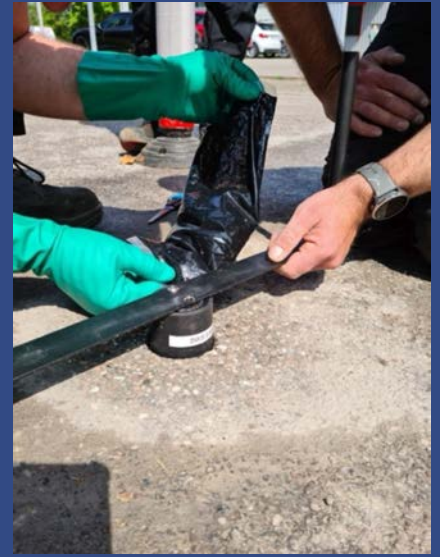
Vergießen des Systems mit Spezial-Harz
